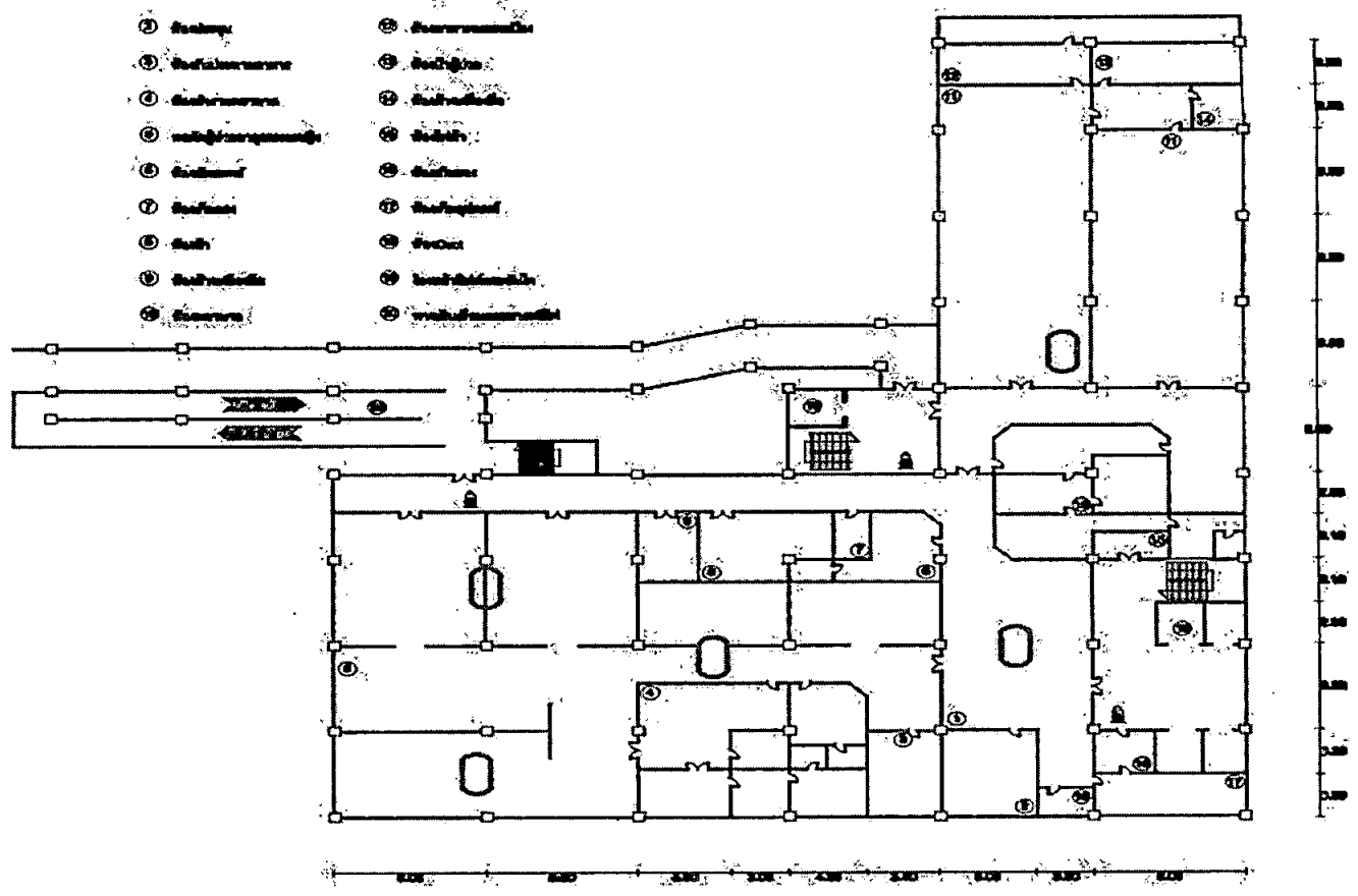
ชั้นที่ 4
